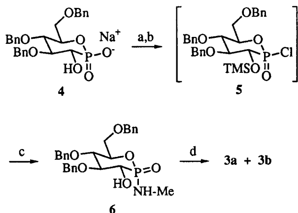
Scheme 1. Synthesis of a phosphonamidate analogue of glucose. a. TMS-OTf, Et 3 N, CH 2 Cl 2 ; b. (COCl) 2 , DMF, CH 2 Cl 2 ; c. CH 3 NH 2 , CH 2 Cl 2 ; d. H 2 , PtO 2 , CH 3 OH, 1500 psi.
